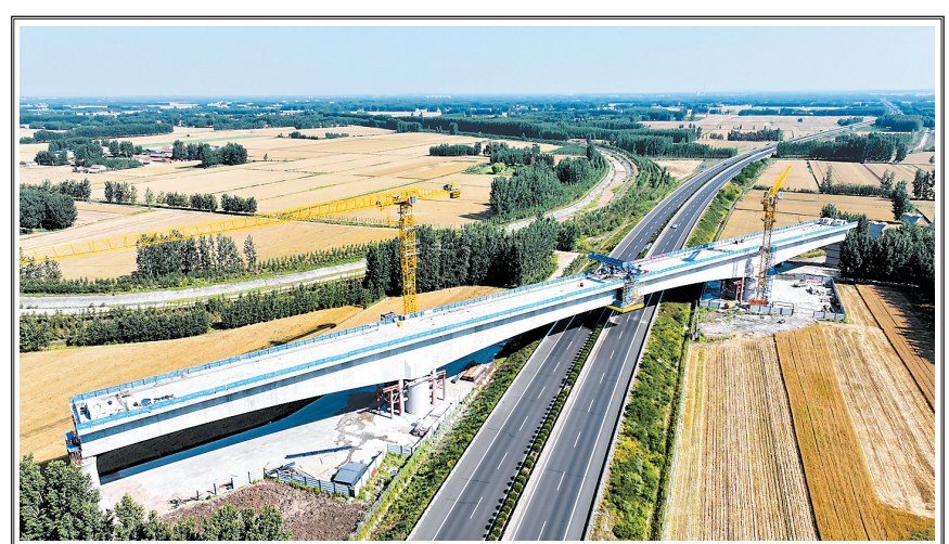
潍宿高铁跨潍日高速连续梁顺利合龙 6月11日,由雄安高速铁路有限公司建设、中铁十一局承建的潍(坊)宿(迁)高铁诸城潍河特大桥跨潍(坊)日(照)高速连续梁顺利合龙,为后续各项施工奠定基础。 新华社记者 郭绪雷 摄
