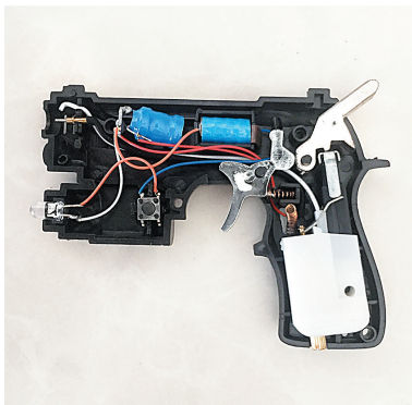
电人玩具枪内部结构
